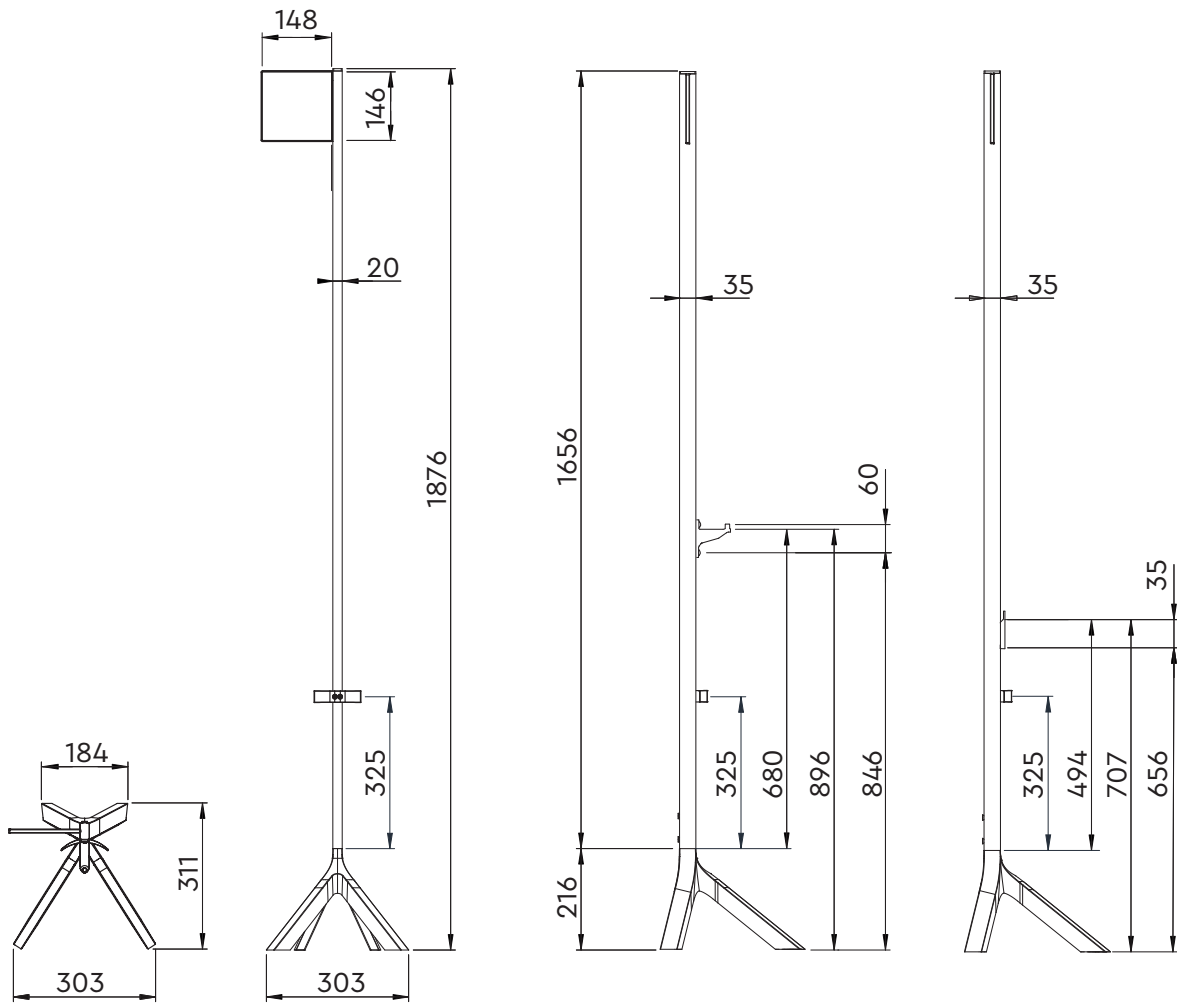
DISEGNO TECNICO 85203 / TECHNICAL DRAWING 85203
