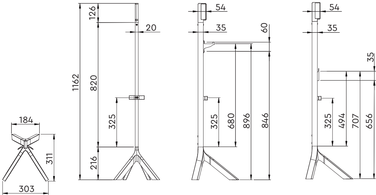
DISEGNO TECNICO 85200 / TECHNICAL DRAWING 85200
